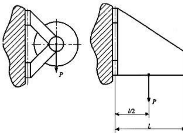
Рисунок 1 - Схема приложения нагрузки к рукавной кассете
